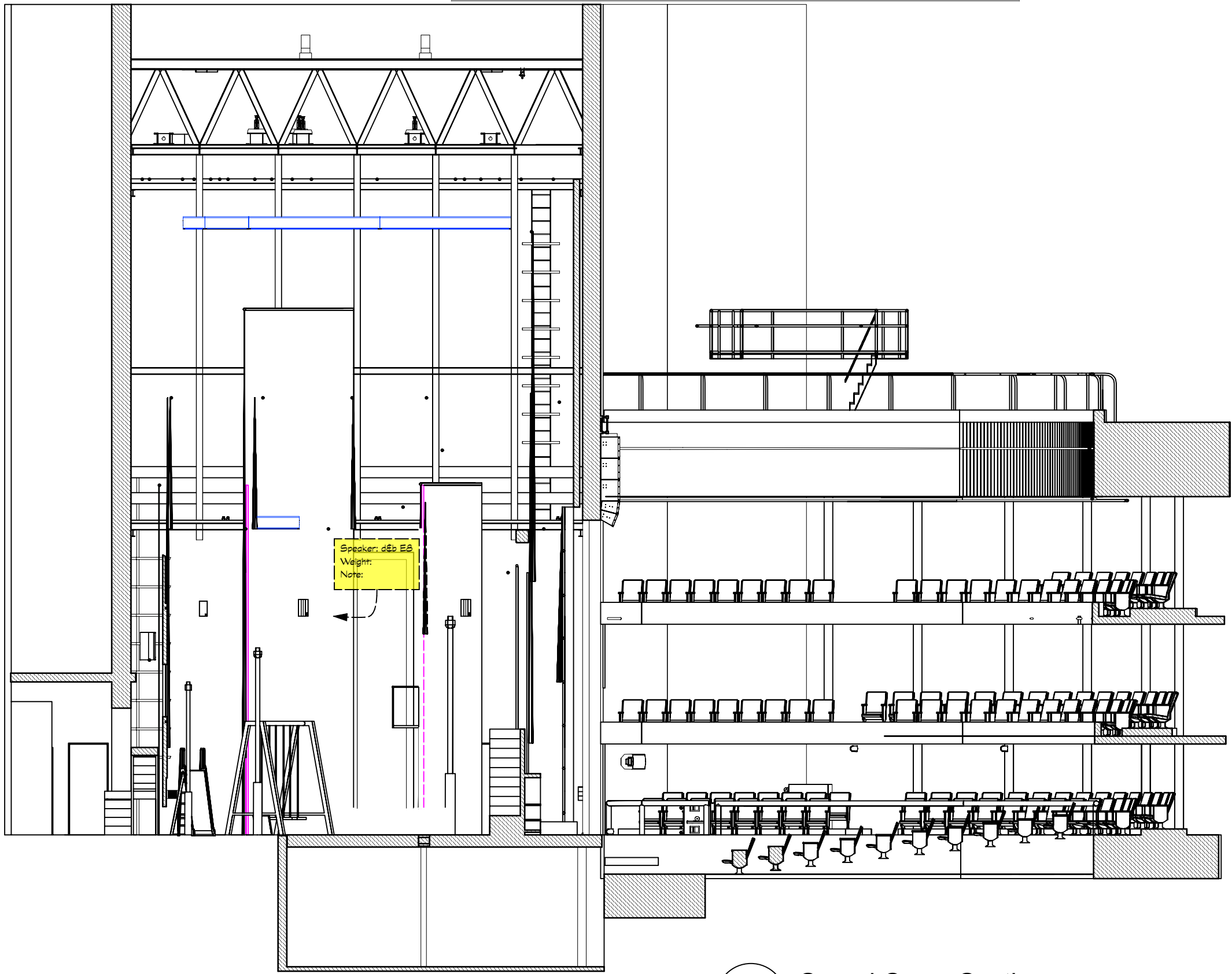
001 Sound Cross Section Scale: 1:100
