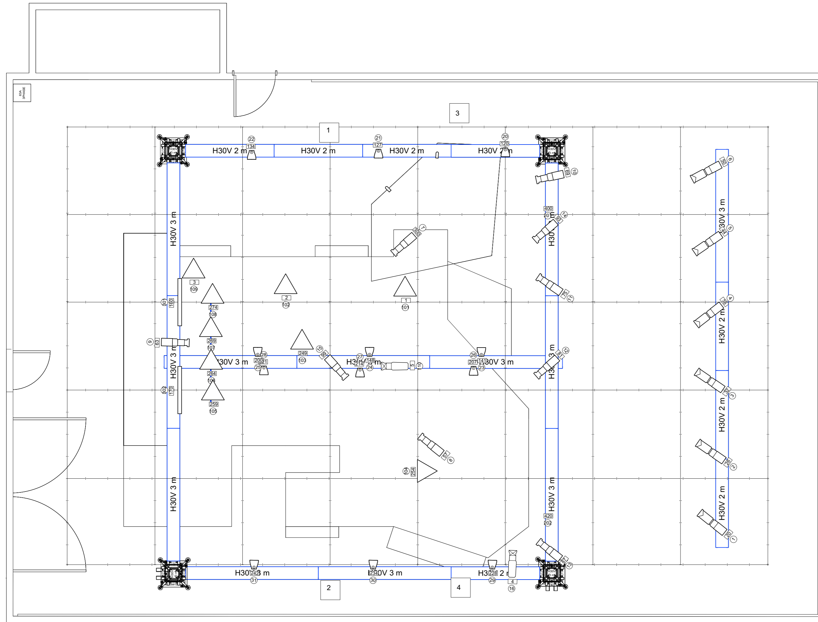
1 LX Plan - The Coat Scale: 1:50
