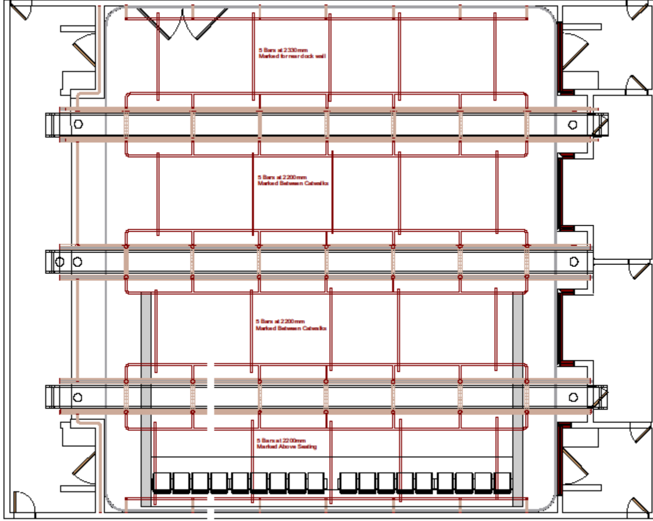
Scale: 1:75 Chandler Crossbars Default Setup
