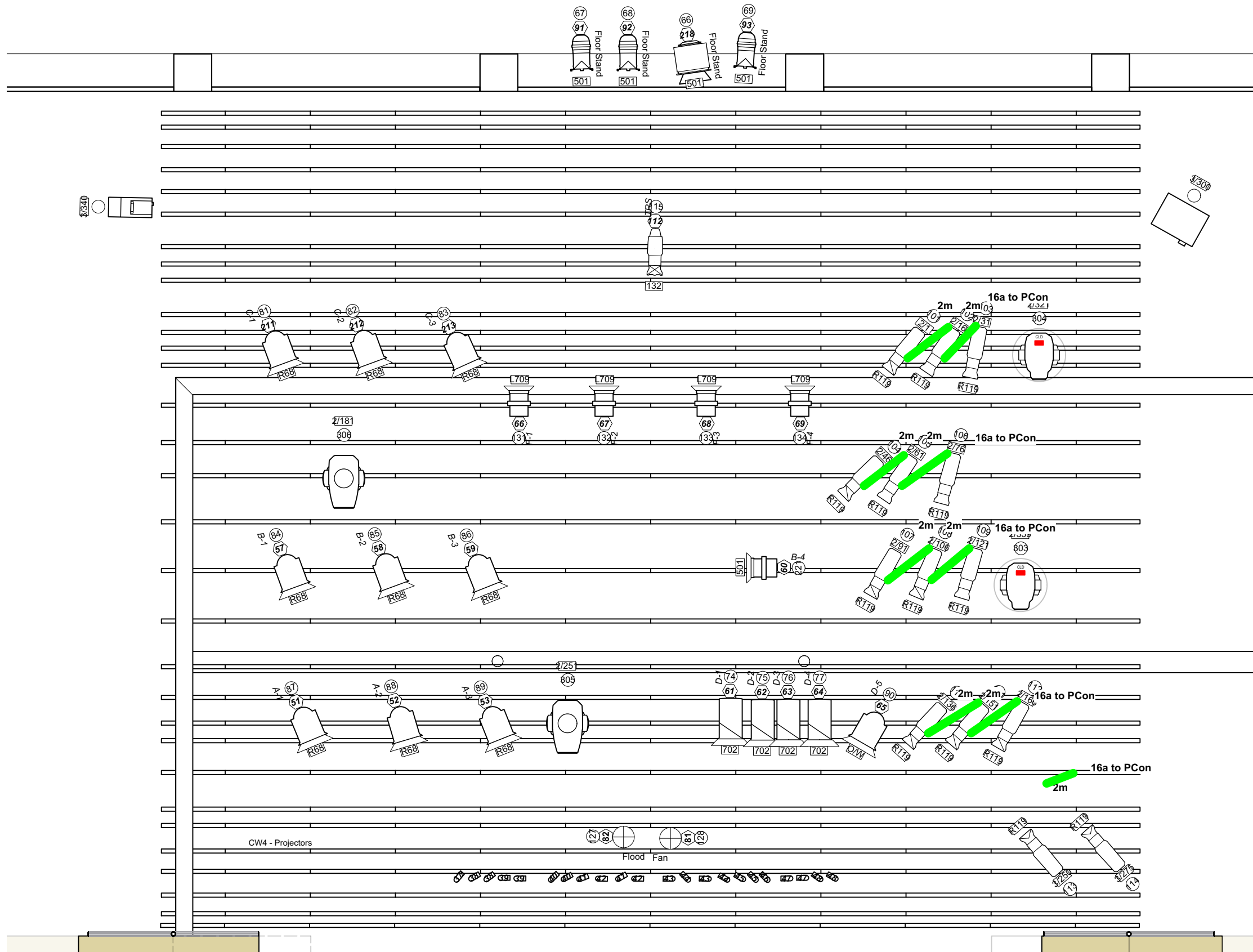
1 PCon Overhead Scale: 1:50
