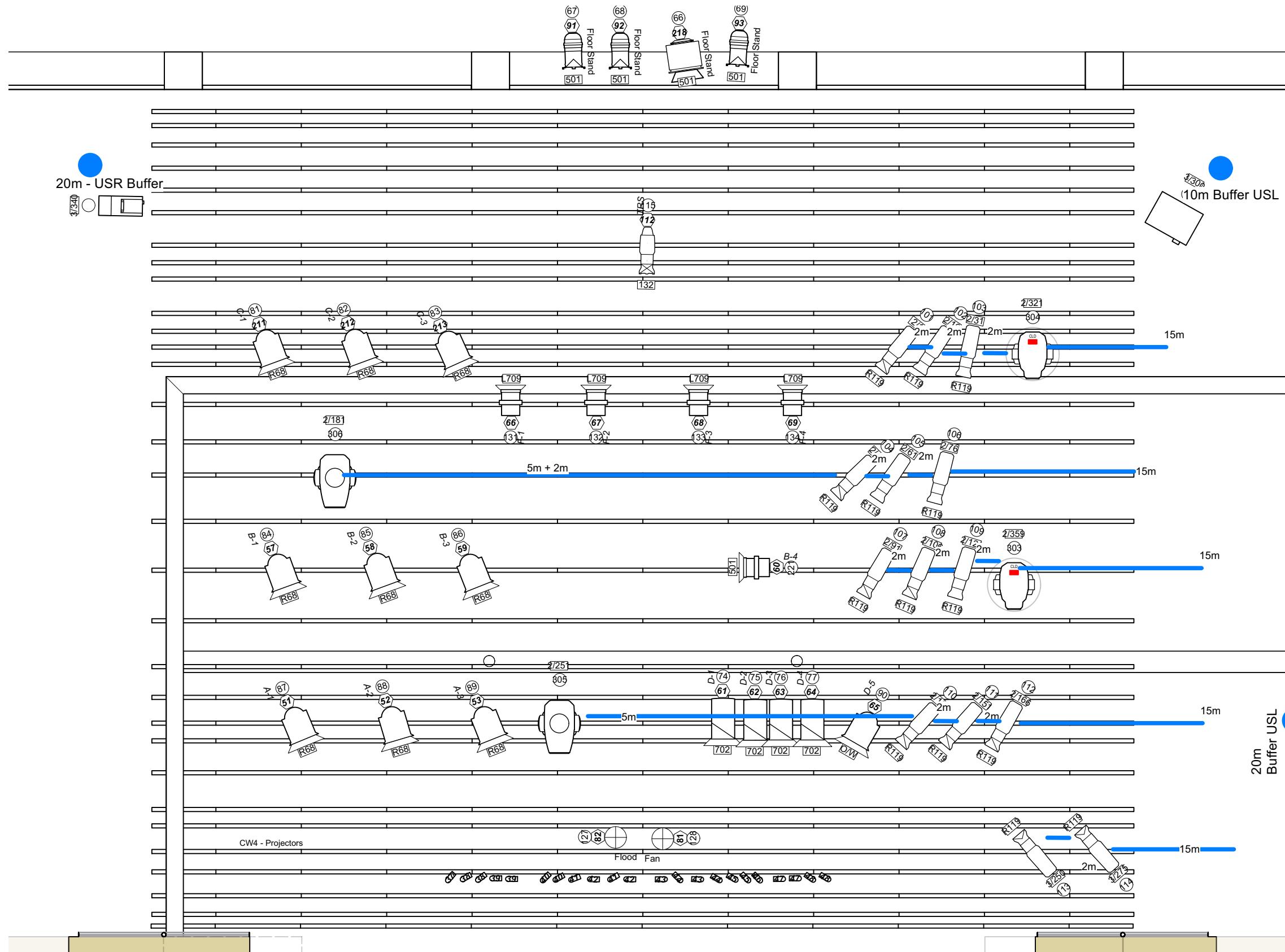
1 DMX Overhead - Dissocia Scale: 1:50
