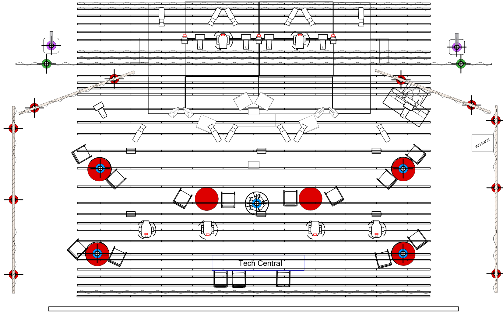
1 A4 Ground Plan Scale: 1:75
